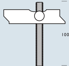
FXTB TOGGLE BOLT M.C.H Ø23
